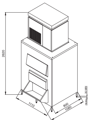
BIN 1200 DD - SM 750/1300
