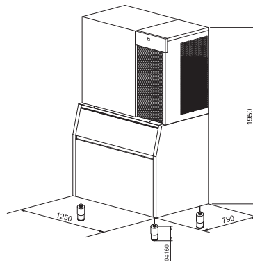
BIN T 830 - CV 1650
