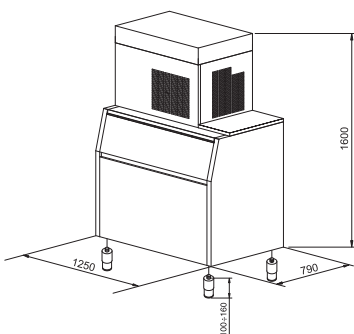
BIN T 830 - SM 500
