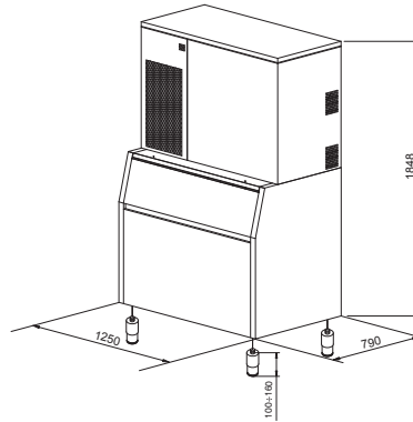
BIN T 830 - CM 650
