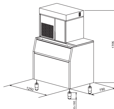
BIN T 830 - SM 750 - SM 1300
