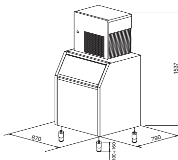
BIN T 420 - GM 330
