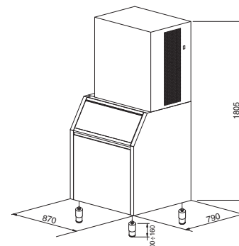
BIN T 420 - CV 475 - CV 950
