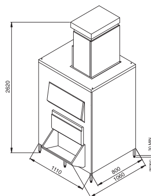
BIN 1200 DD - SPLIT 750/1300
