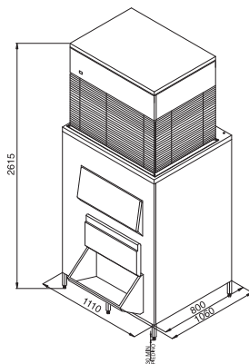
BIN 1200 DD - GM 2000
