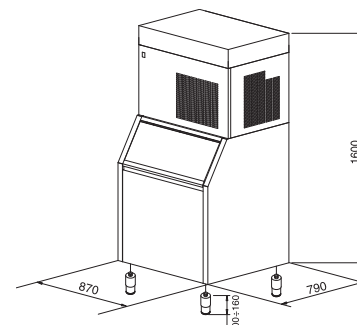
BIN T 420 - SM 500
