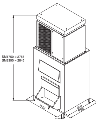
BIN 1200 DD - SM 1750 - SM 3300
