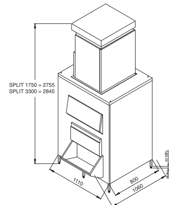
BIN 1200 DD - SPLIT 1750/3300
